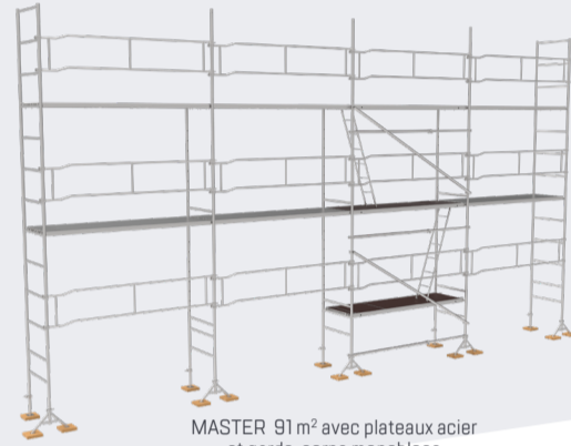
MASTER 91 m 2 avec plateaux acier et garde-corps monoblocs
