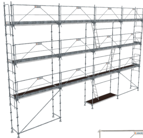
R200 MEDIUM 104 M 2 ACIER avec garde-corps FUSIO
