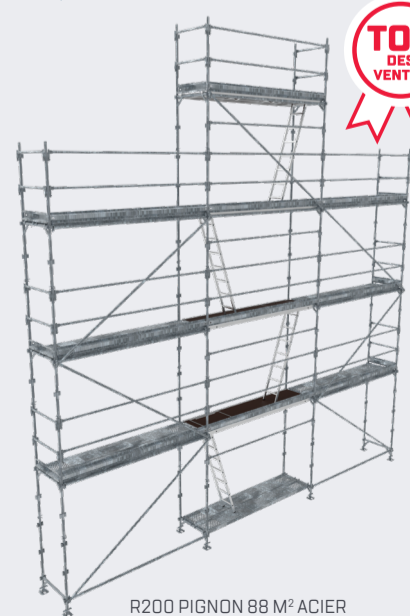
R200 PIGNON 88 M 2 ACIER avec garde-corps lisses et planchers RCE acier
