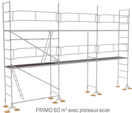
PRIMO 60 m 2 avec plateaux acier et garde-corps monoblocs
