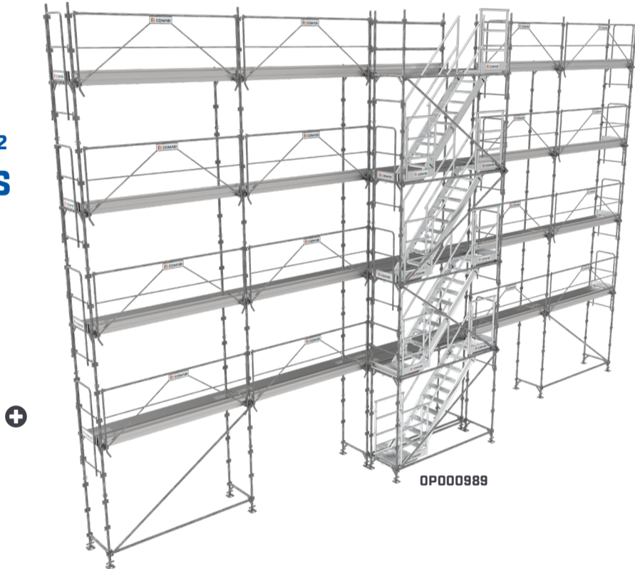
Plancher alu/bois
